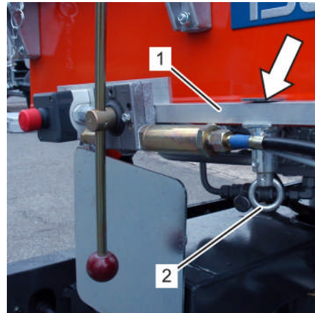
Fig. 117: Télécommande mécanique
