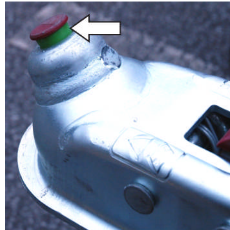
Fig. 72: Vérifier l'indicateur d'usure
