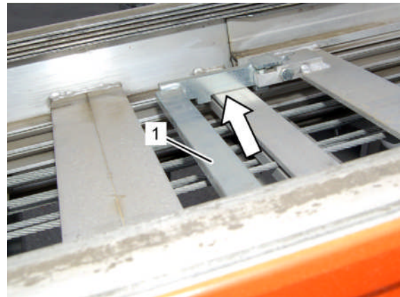
Fig. 248: Verrouillage du rail télescopique
