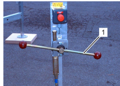
Fig. 249: Levier de manoeuvre du chariot
