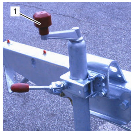
Fig. 89: Abaisser la roue d'appui à la manivelle
