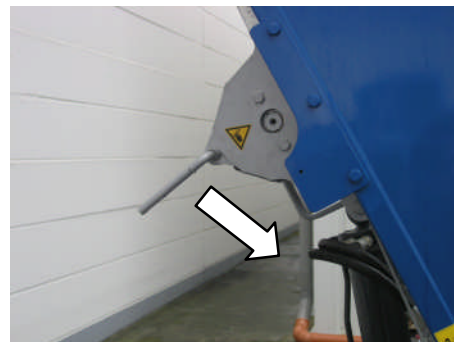
Fig. 251: Blocage à cliquet
