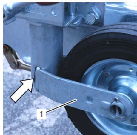
Fig. 76: Point de butée de la roue d'appui
