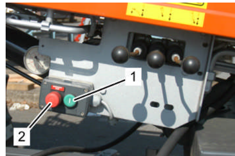
Fig. 135: Démarrage du moteur électrique
