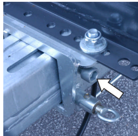
Fig. 44: Serrer le boulon
