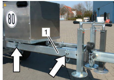
Fig. 104: Sécurisation des appuis
