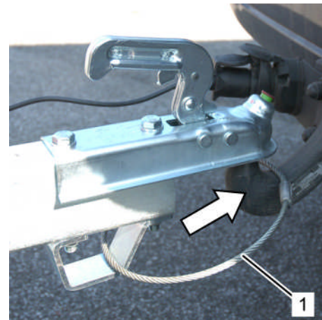
Fig. 92: Retirer le câble de rupture d'attelage
