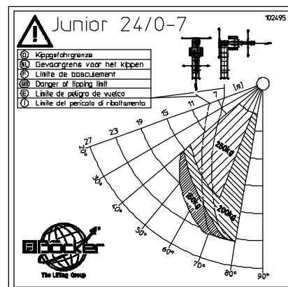
Fig. 140: Tableau de charge
