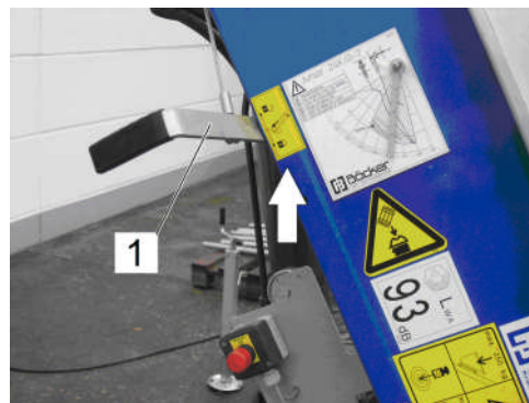
Fig. 201: Blocage du levier du pack de rails
