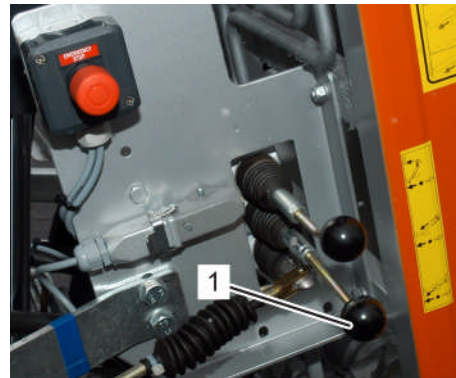
Fig. 256: Rentrer le pack de rails
