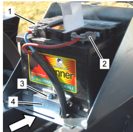
Fig. 291: Déconnecter la batterie
