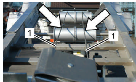
Fig. 187: Poser les câbles à plat
