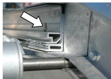
Fig. 174: Mise en place des vis
