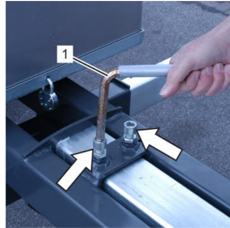
Fig. 245: Boulons du timon télescopique
