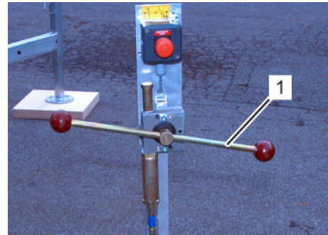
Fig. 166: Levier de manoeuvre du chariot
