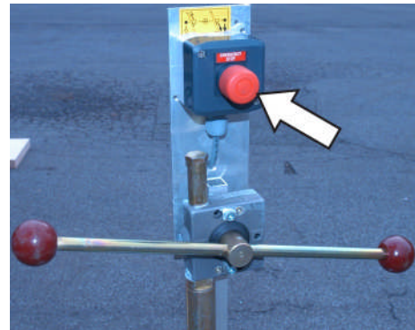
Fig. 24: Interrupteur ARRÊT D'URGENCE
