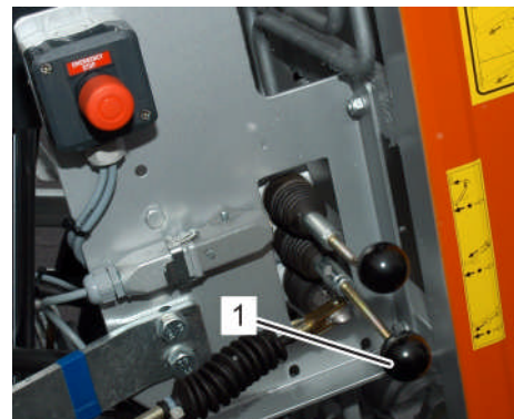
Fig. 149: Déploiement du pack de rails
