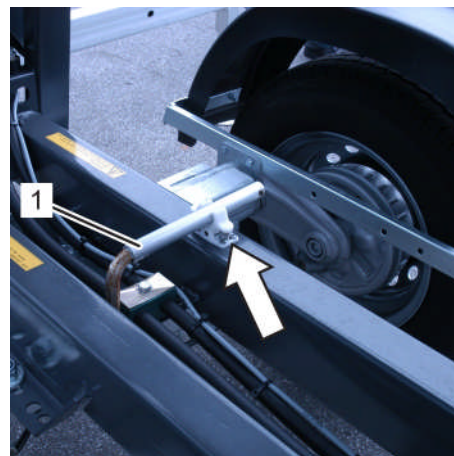
Fig. 232: Retirer la clé de son logement
