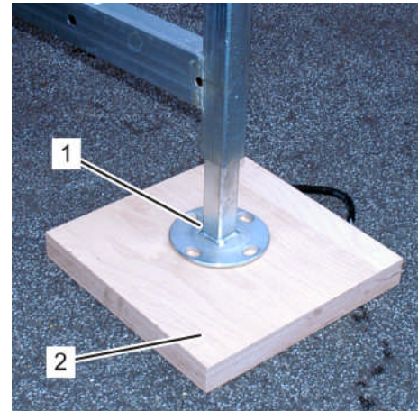
Fig. 109: Placer une cale sous les appuis
