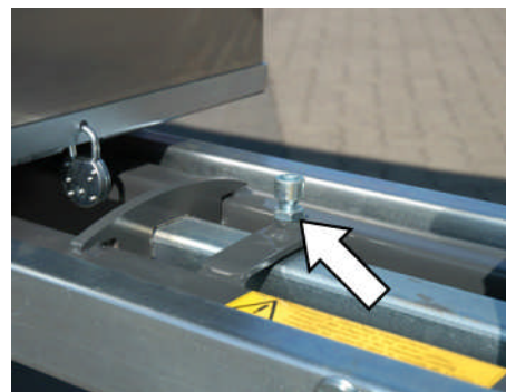
Fig. 50: Boulon de l'essieu télescopique
