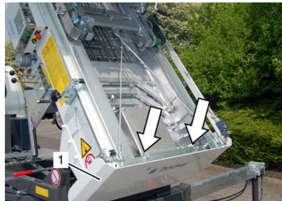
Fig. 67: tôle de terminaison
