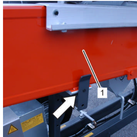
Fig. 35: Vérifier la position du pack de rails
