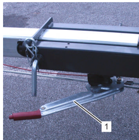
Fig. 84: Serrer le frein à main.
