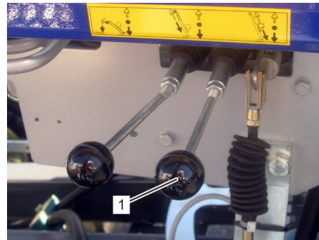
Fig. 250: Rentrer le pack de rails
