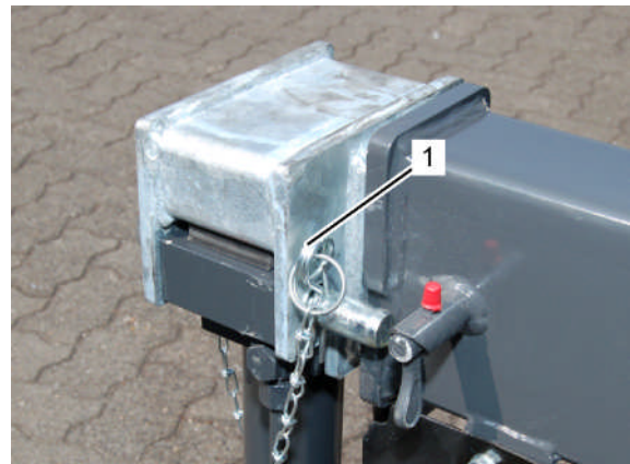
Fig. 276: Retirer la goupille de sécurité
