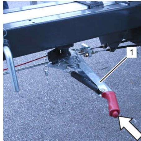
Fig. 83: Desserrer le frein à main (Exemple)
