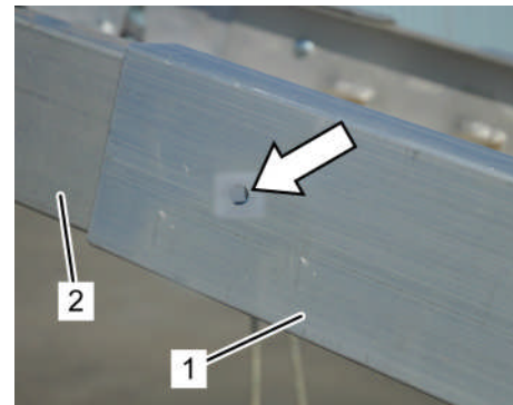
Fig. 193: Mettre en place la bride extérieure
