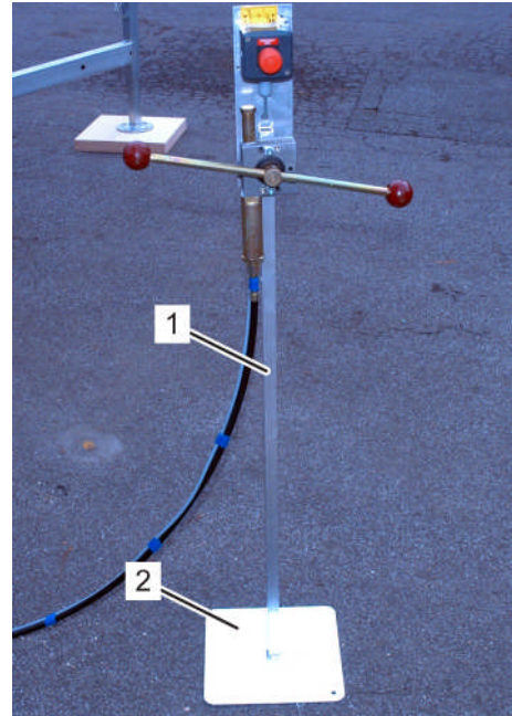
Fig. 298: Télécommande mécanique
