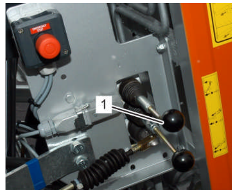
Fig. 153: Levier de commande Réglage angulaire
