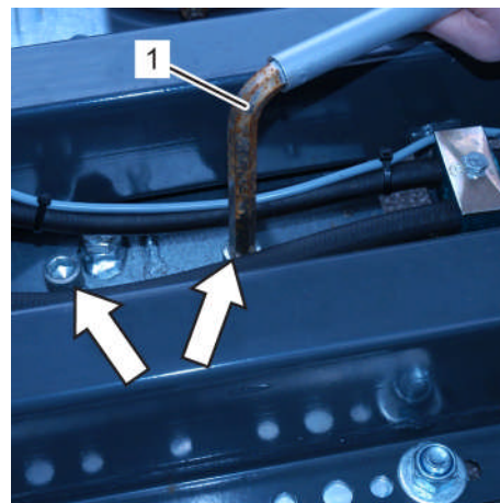
Fig. 226: Boulons de l'essieu télescopique
