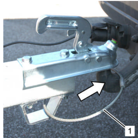
Fig. 74: Câble de rupture d'attelage
