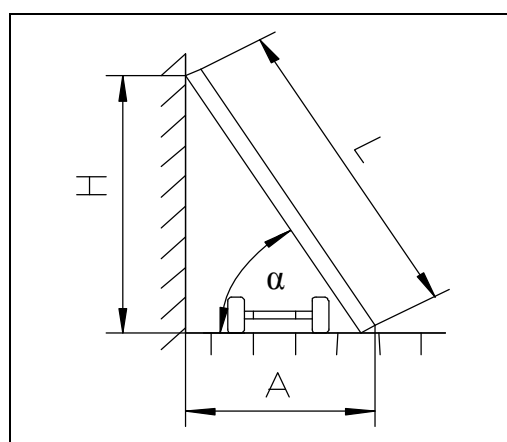
Fig. 97: Hauteurs atteintes sur le bâtiment
