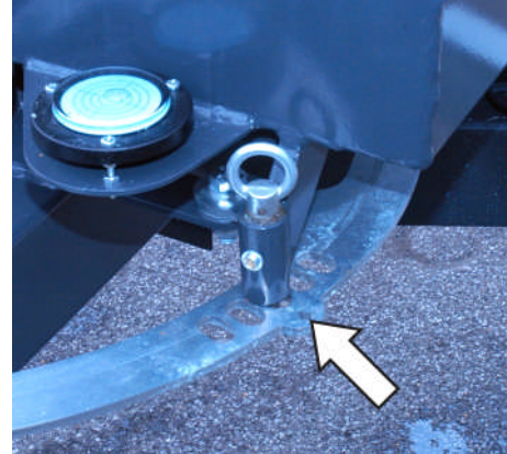
Fig. 258: Position de base sur la tôle à alésages.
