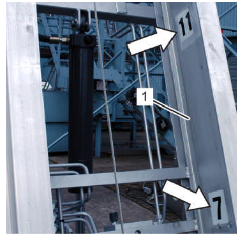
Fig. 148: Lecture de la hauteur de déploiement des rails
