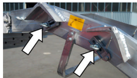
Fig. 178: Réglage du déflecteur
