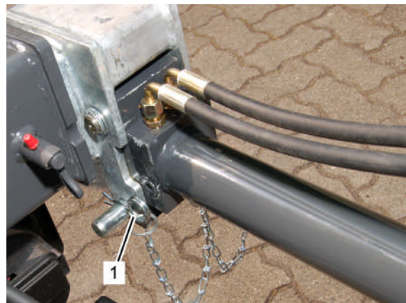
Fig. 279: Mettre en place la goupille
