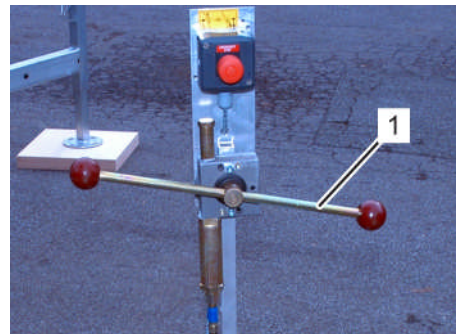
Fig. 246: Levier de manoeuvre du chariot
