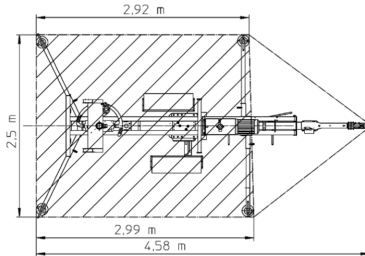
Fig. 95: Surface d'appui d'un appareil freiné avec timon rentré en m
