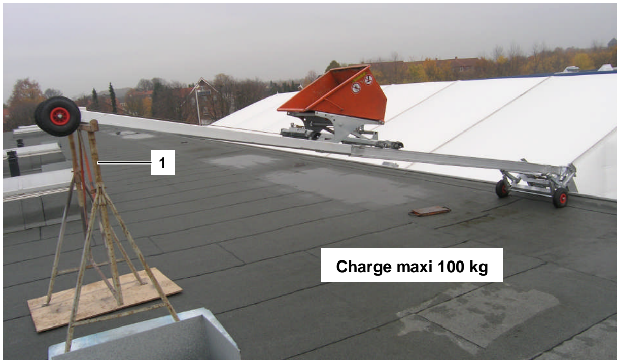
Fig. 213: Charge et appui à une charge de 100 kg
