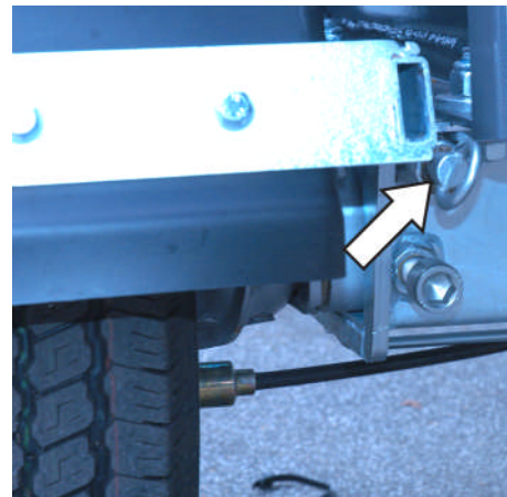
Fig. 235: Clavette de l'essieu télescopique
