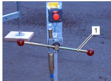
Fig. 253: Levier de manoeuvre du chariot
