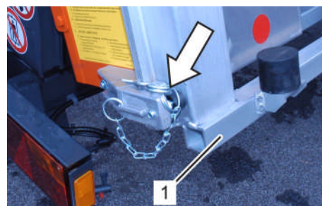
Fig. 156: Rail inférieur de prolongation
