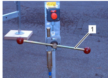
Fig. 168: Levier de manoeuvre du chariot
