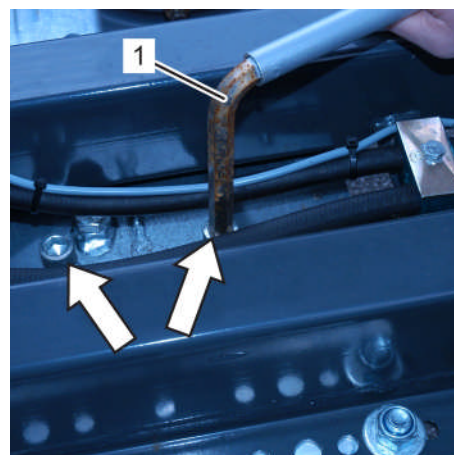
Fig. 233: Boulons de l'essieu télescopique
