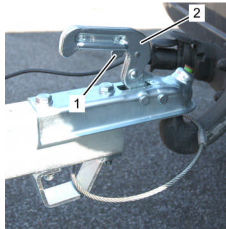
Fig. 93: Desserrer le verrouillage
