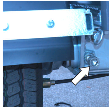
Fig. 236: Boulons de l'essieu télescopique
