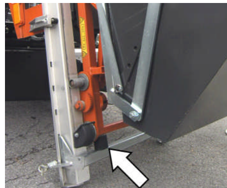
Fig. 165: Ramener le chariot sur ses butoirs en caoutchouc
