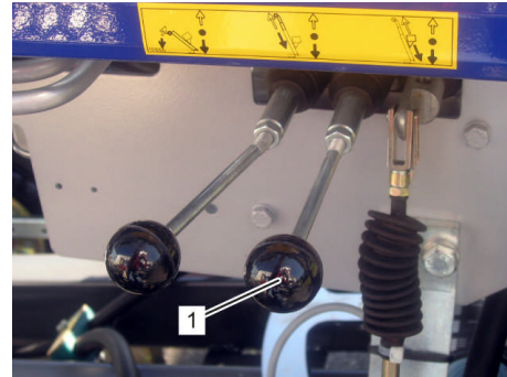
Fig. 203: Déploiement du pack de rails
