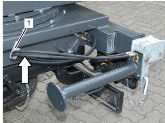
Fig. 63: vérifier les conduites hydrauliques
