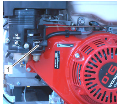
Fig. 263: Fermer le robinet d'essence
