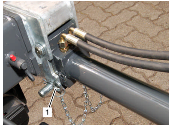
Fig. 61: vérifier la goupille de sécurité
