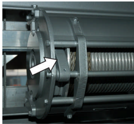
Fig. 150: Blocage à cliquet
