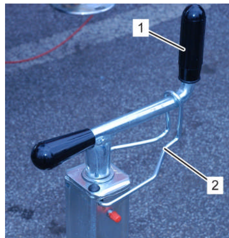
Fig. 274: Sécurisation des manivelles
