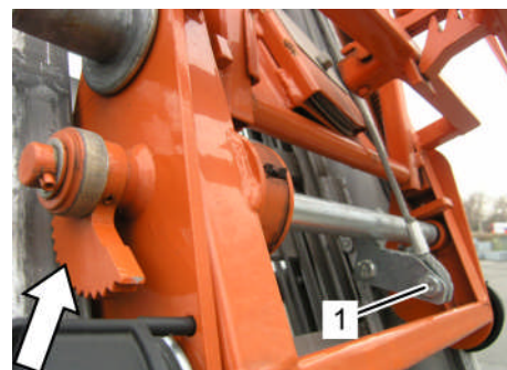
Fig. 284: Vérifier les attaches de câbles
