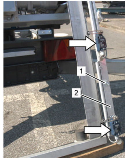
Fig. 158: Interrupteur du point de freinage et d'arrêt
