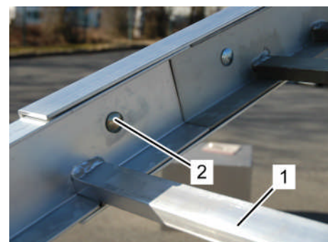
Fig. 195: Vérifier la surface de positionnement
