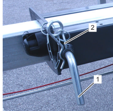
Fig. 244: Boulon du timon télescopique
