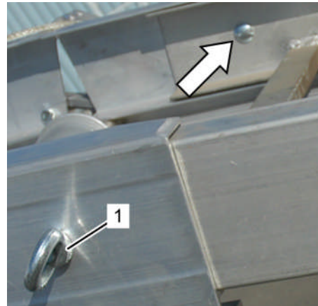
Fig. 189: Monter la pièce faitière
