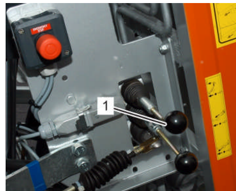
Fig. 255: Levier de commande Réglage angulaire
