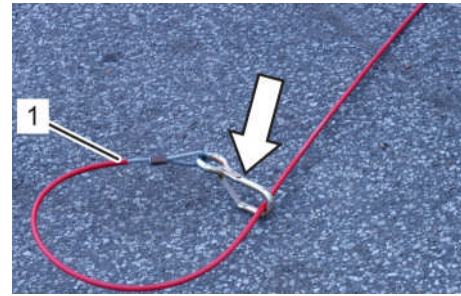
Fig. 90: Câble de rupture d'attelage du frein d'inertie
