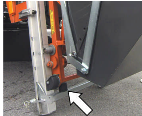
Fig. 283: Abaisser le chariot
