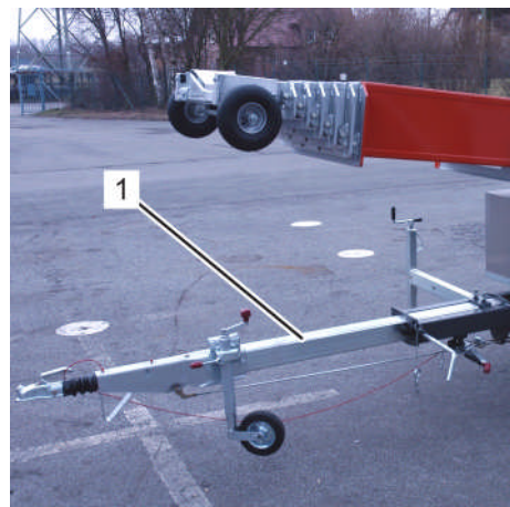
Fig. 46: Timon télescopique
