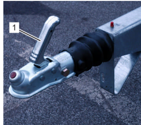
Fig. 69: Défaire le verrouillage
