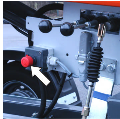
Fig. 23: Interrupteur ARRÊT D'URGENCE
