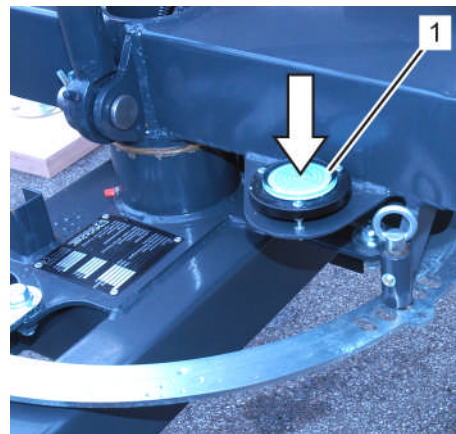
Fig. 112: Niveau à bulle
