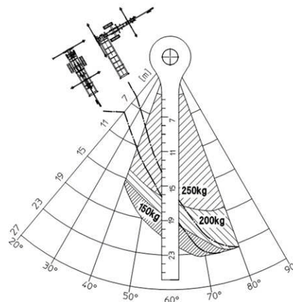
Fig. 257: Tableau de charge
