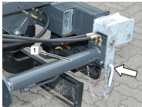
Fig. 60: vérifier les appuis arrière
