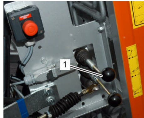
Fig. 161: Levier de commande Réglage angulaire
