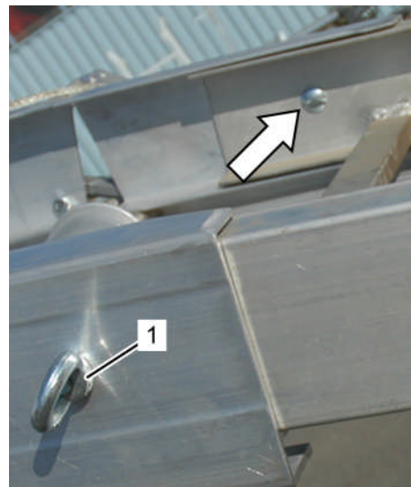
Fig. 185: Serrage des boulons du prolongateur de rail
