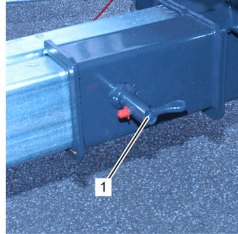
Fig. 103: Enclencher les appuis avant
