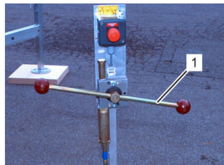
Fig. 190: Levier de manoeuvre du chariot
