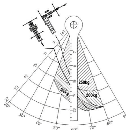
Fig. 162: Tableau de charge
