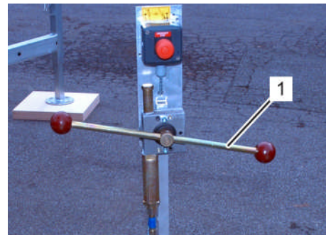
Fig. 216: Levier de manoeuvre du chariot
