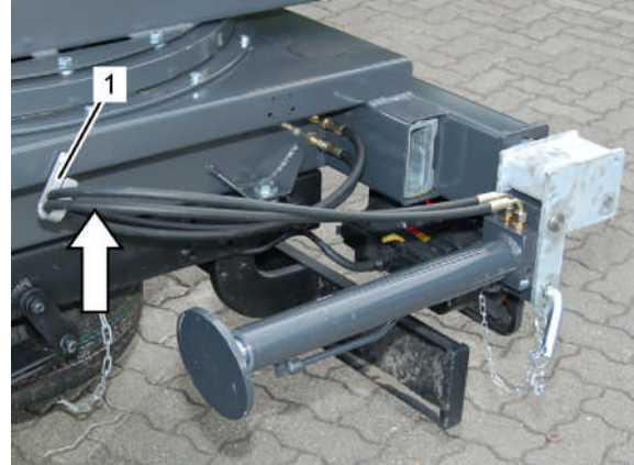
Fig. 280: Accrocher les conduites hydrauliques
