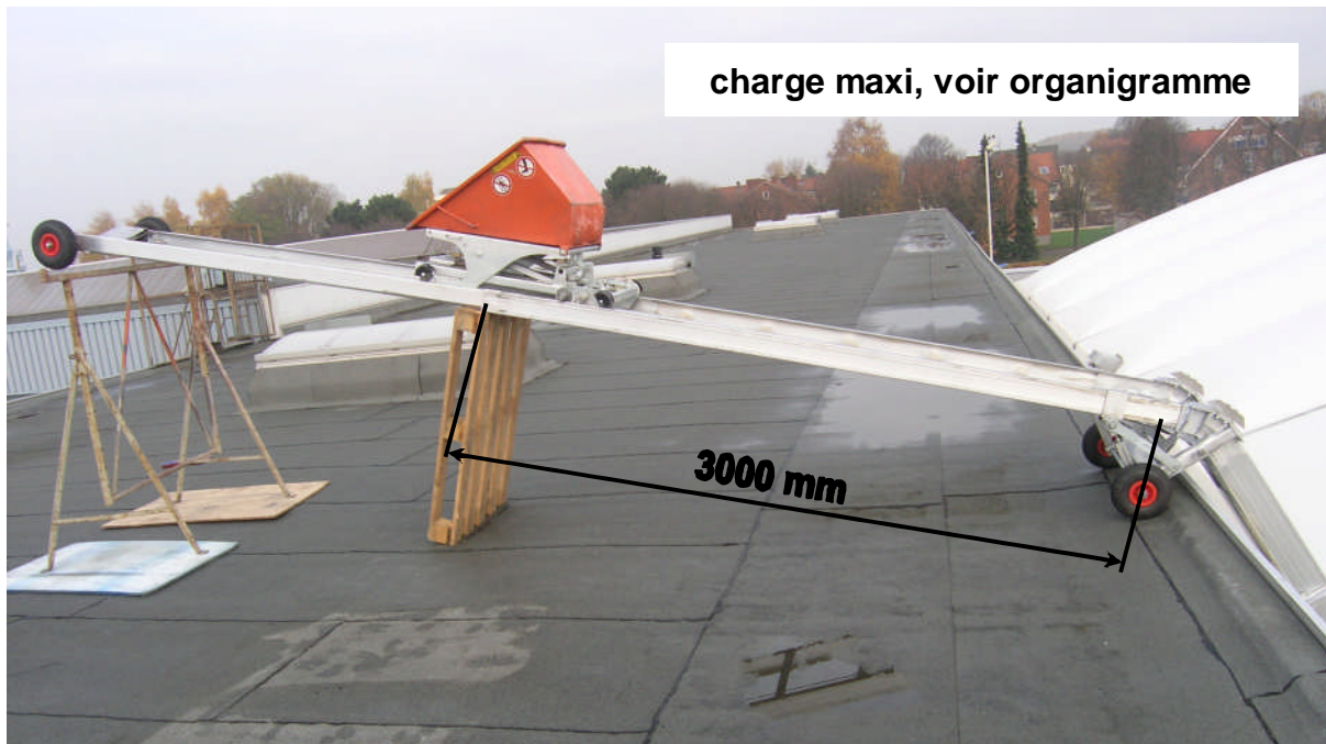
Fig. 212: Charge et appui à la charge maxi
