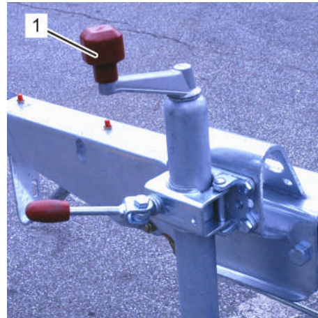
Fig. 111: Libérer la roue d'appui
