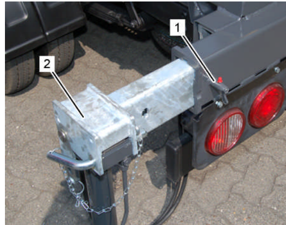
Fig. 275: Rentrer l'appui
