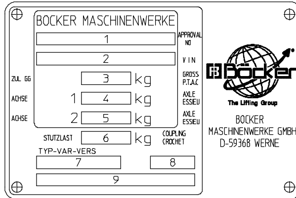
Fig. 29: Plaque signalétique de la remorque
