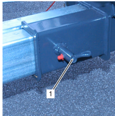
Fig. 101: Déverrouiller les béquilles d'appui avant
