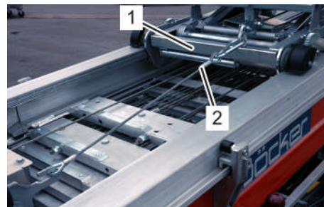
Fig. 36: Câble d'arrimage
