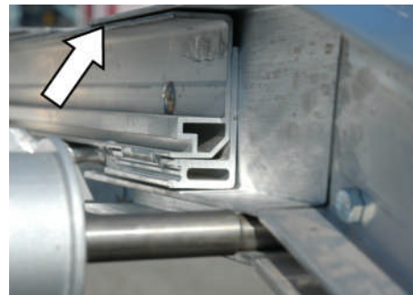
Fig. 176: Contrôle du déflecteur
