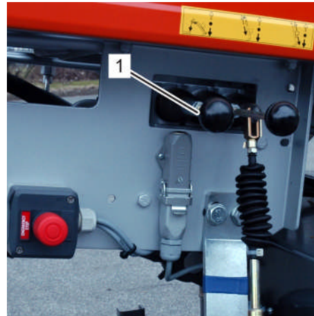
Fig. 141: Levier de commande Réglage angulaire
