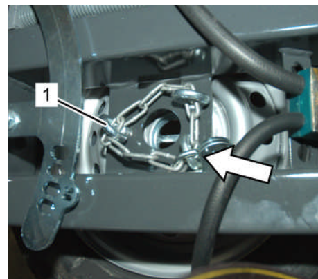
Fig. 293: Chaîne de sécurité de la roue de secours
