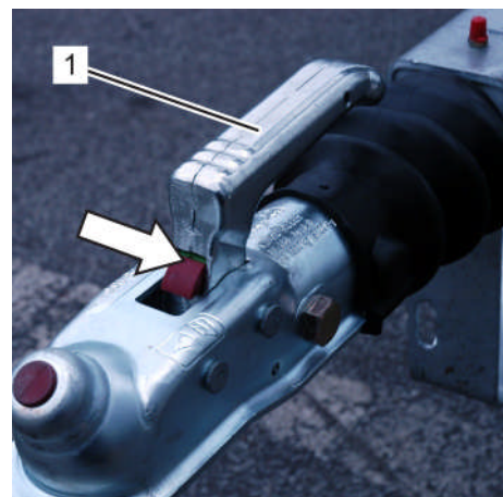
Fig. 71: Mettre le verrouillage en tension
