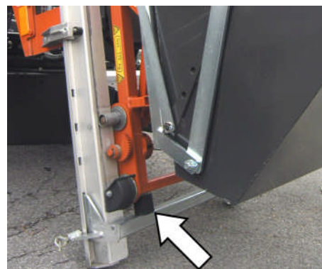
Fig. 159: Ramener le chariot sur ses butoirs en caoutchouc
