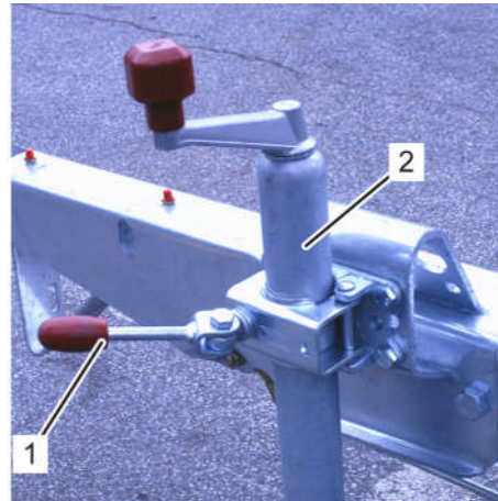
Fig. 77: Relever la roue d'appui
