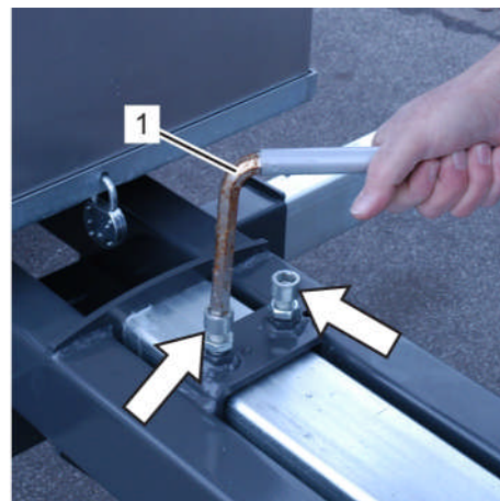
Fig. 49: Boulons de l'essieu télescopique
