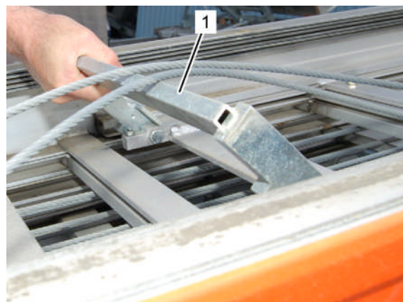
Fig. 207: Verrouillage rail articulé
