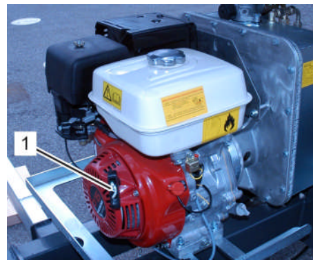
Fig. 127: Câble de lancement du moteur
