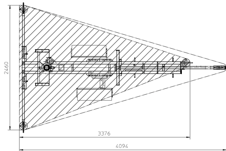
Fig. 96: Surface d'appui d'un appareil non freiné avec timon rentré en mm
