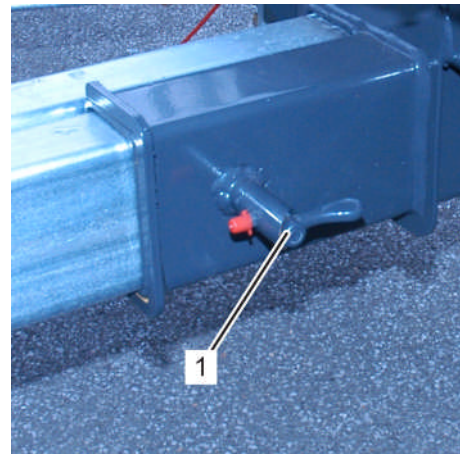
Fig. 271: Déverrouiller les fixations arrière
