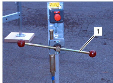
Fig. 206: Levier de manoeuvre du chariot
