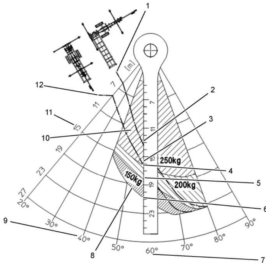
Fig. 211: Exemple de lecture du tableau de charge
