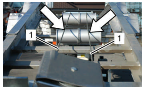
Fig. 191: Vérifier les câbles
