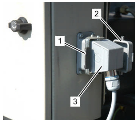
Fig. 217: Prise de la télécommande
