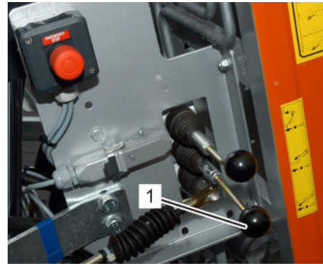
Fig. 147: Déploiement du pack de rails
