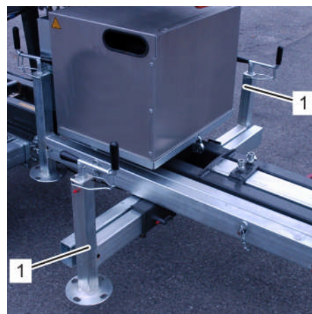
Fig. 102: Tirer les appuis avant vers l'extérieur
