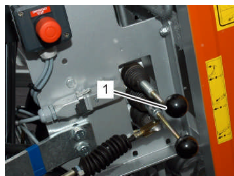
Fig. 155: Levier de commande Réglage angulaire
