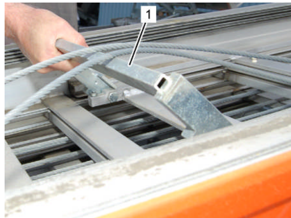
Fig. 247: Verrouillage du rail télescopique
