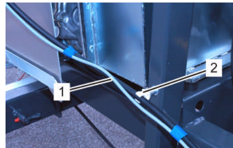
Fig. 120: Fixation du câble
