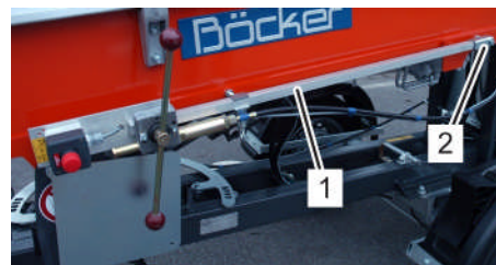
Fig. 64: Vérification de la télécommande
