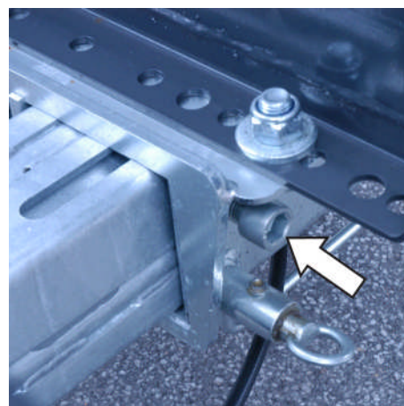
Fig. 227: Serrer le boulon
