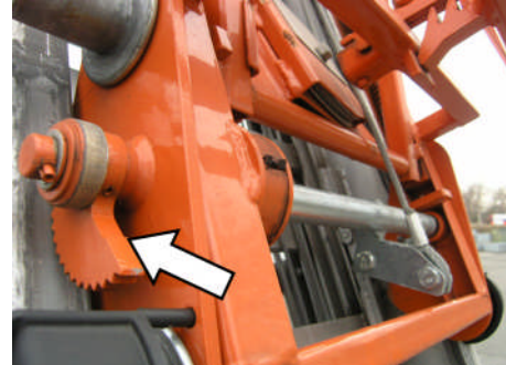
Fig. 287: Vérifier le dispositif de retenue
