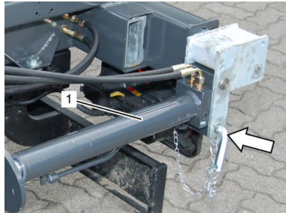
Fig. 278: Mettre en place le boulon
