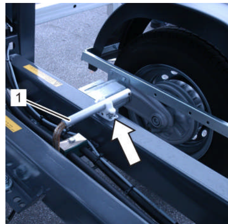
Fig. 240: Retirer la clé de son logement
