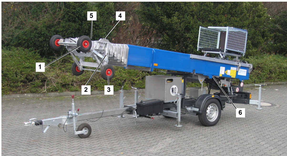
Fig. 34: Vue d'ensemble de la version HD 24K/0-7 avec déflecteur
