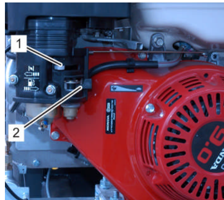
Fig. 126: Levier de starter
