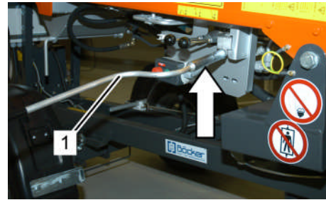
Fig. 215: Levier de manoeuvre du chariot
