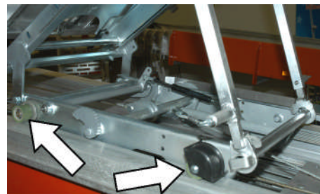
Fig. 282: Chariot
