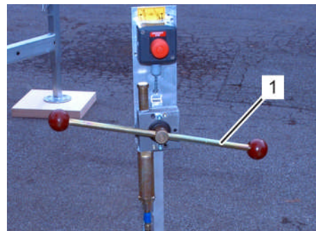
Fig. 200: Levier de manoeuvre du chariot
