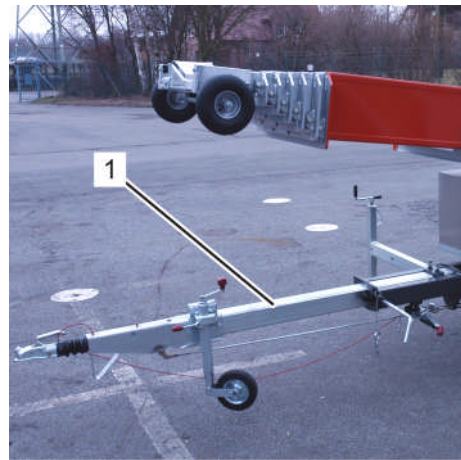
Fig. 239: Timon télescopique
