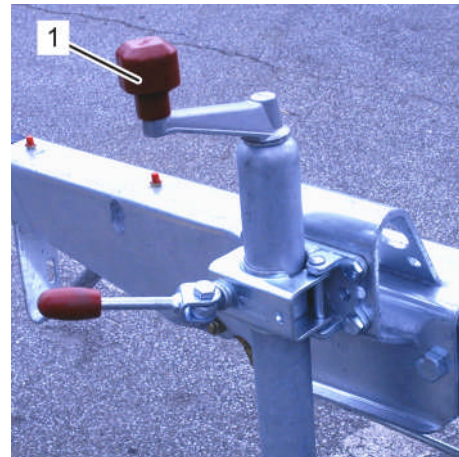
Fig. 75: Relever à la manivelle la roue d'appui
