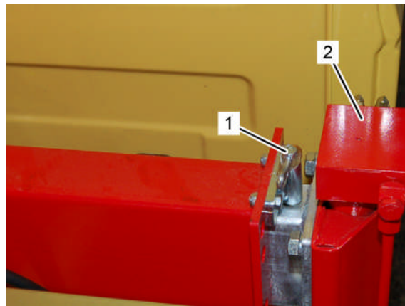
Fig. 59: vérifier les appuis avant
