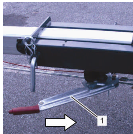
Fig. 98: Serrer le frein à main.
