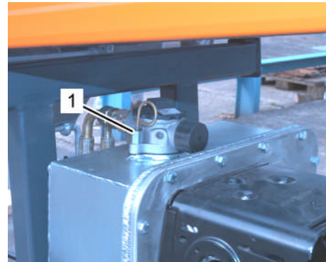
Fig. 123: Jauge
