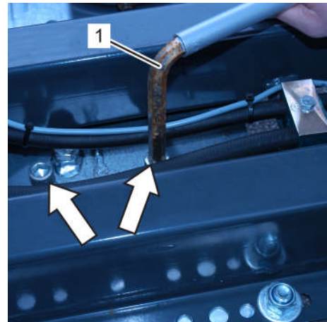
Fig. 229: Boulons de l'essieu télescopique
