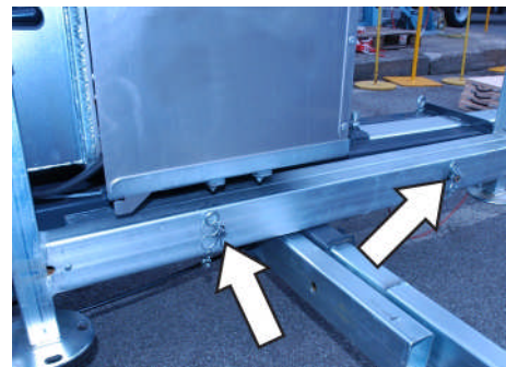
Fig. 105: Sécurisation des appuis
