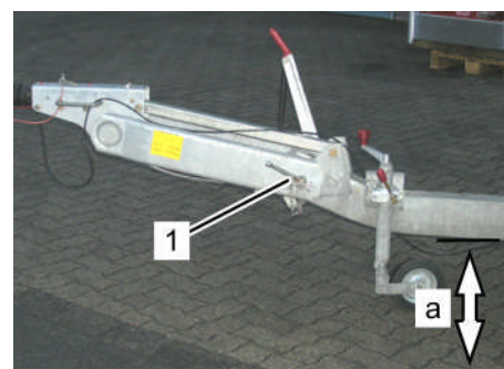
Fig. 78: Timon réglable en hauteur
