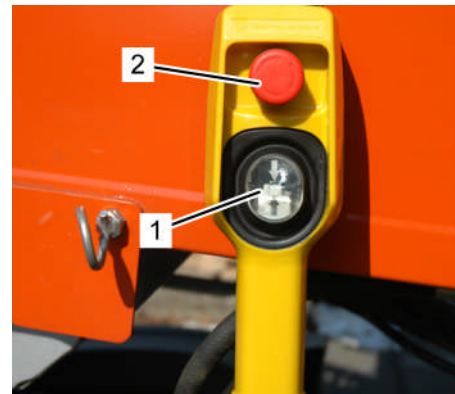
Fig. 218: Télécommande UE
