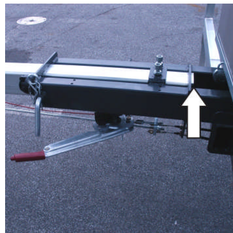
Fig. 243: Vérification du timon télescopique
