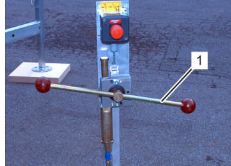
Fig. 137: Levier de manoeuvre du chariot
