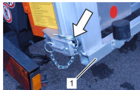
Fig. 254: Prolongateur de rail
