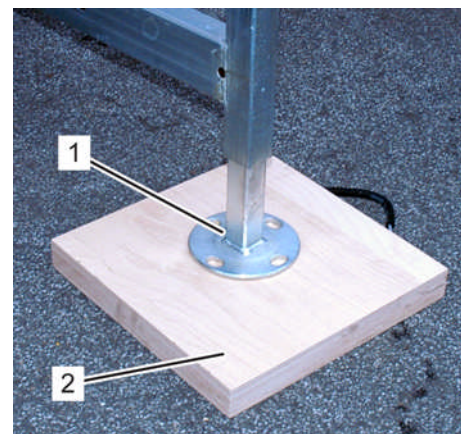
Fig. 99: Placer une cale sous les appuis
