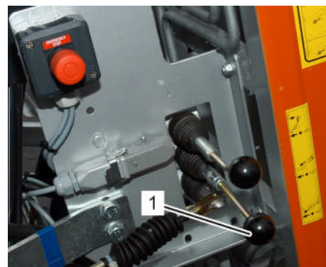
Fig. 182: Déploiement du pack de rails
