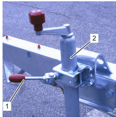
Fig. 88: Abaisser la roue d'appui
