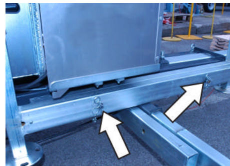
Fig. 272: Sécurisation des appuis
