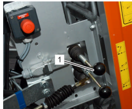
Fig. 180: Levier de commande Réglage angulaire
