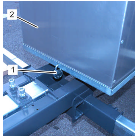
Fig. 122: Retirer le capot du moteur
