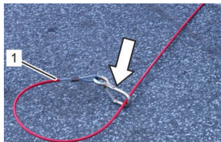
Fig. 73: Câble de rupture d'attelage du frein d'inertie
