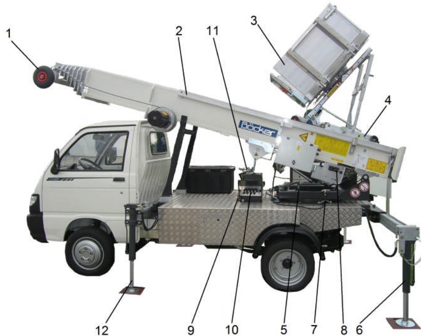
Fig. 33: vue d'ensemble de la structure montée sur camion
